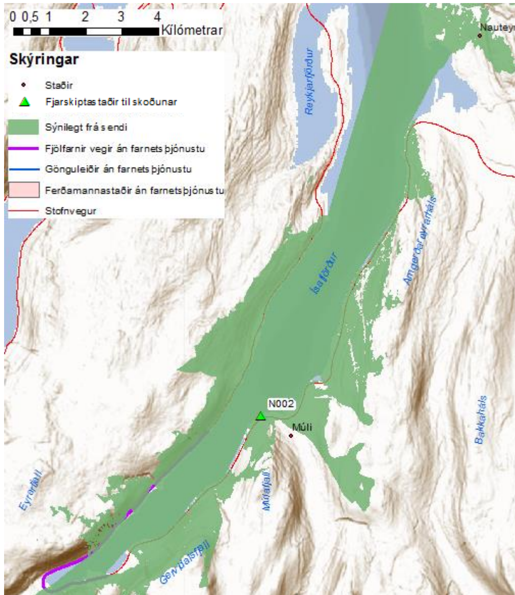
Mynd 10: Sjónlínudreifing frá sendi N002.
