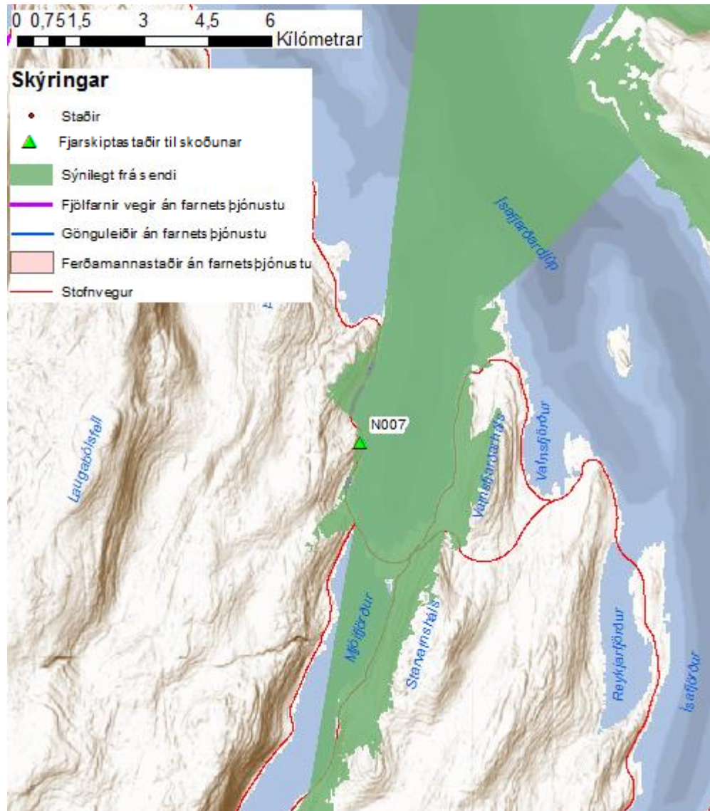
Mynd 8: Sjónlínudreifing frá sendi N007 við Látranúp.
