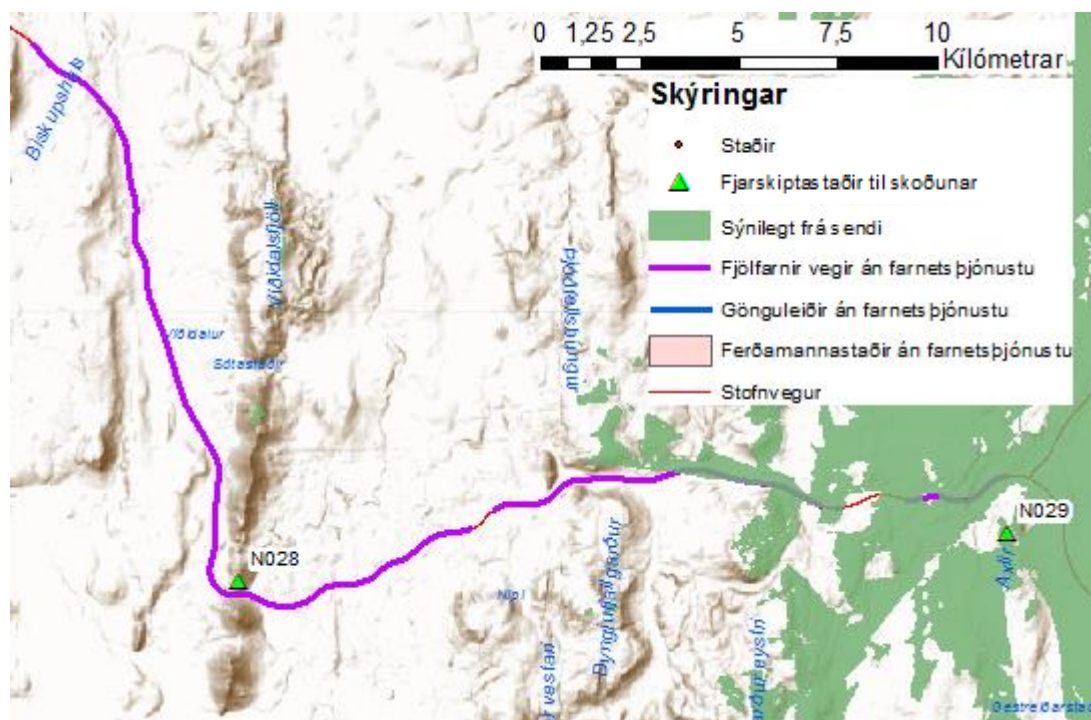
Mynd 44: Sjónlínudreifing frá N029 með 20m mastri.
